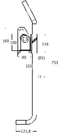
Teknik Resim / Drawing
