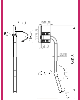
Teknik Resim / Drawing
