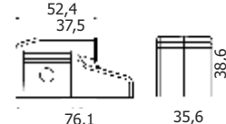
İ-761-10 Sağ / Right
