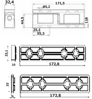
Teknik Resim / Drawing
