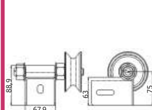
Teknik Resim /Drawing
