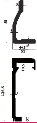
Teknik Resim / Drawing
