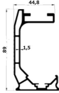
Teknik Resim / Drawing
