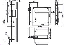
Teknik Resim / Drawing
