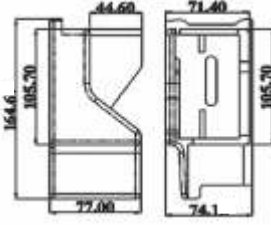
Teknik Resim / Drawing
